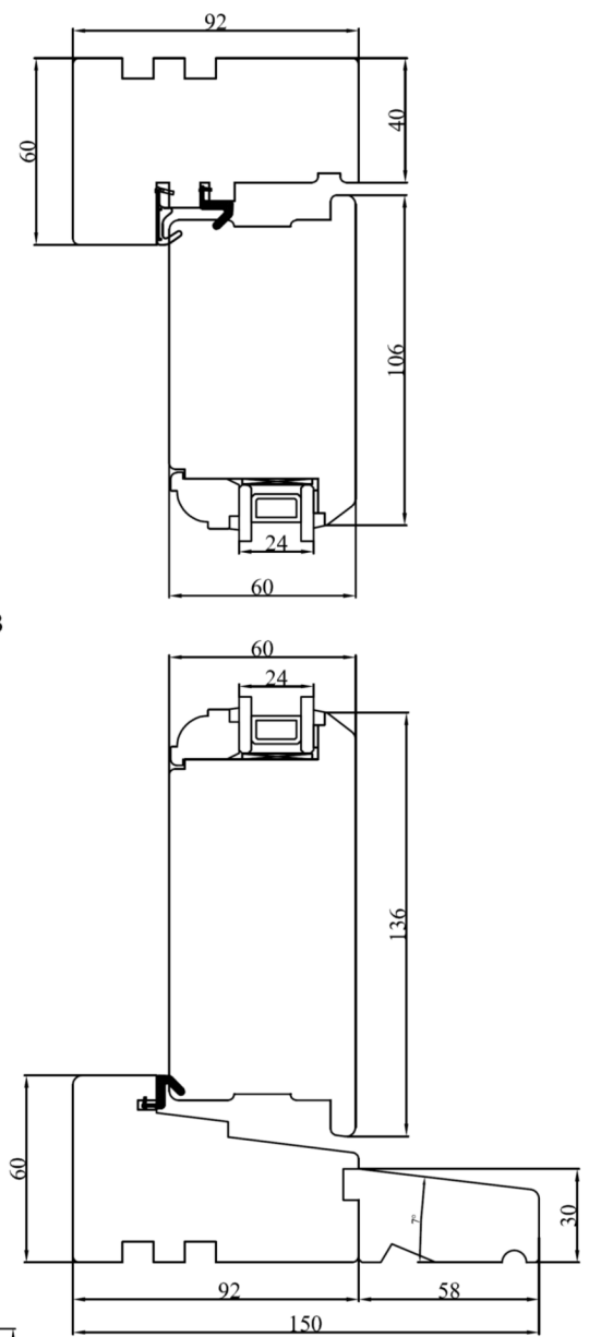
Section A-A
