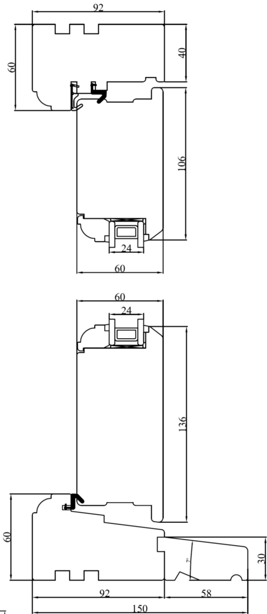
Section A-A
