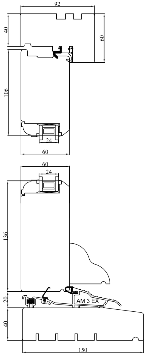
Section A-A
